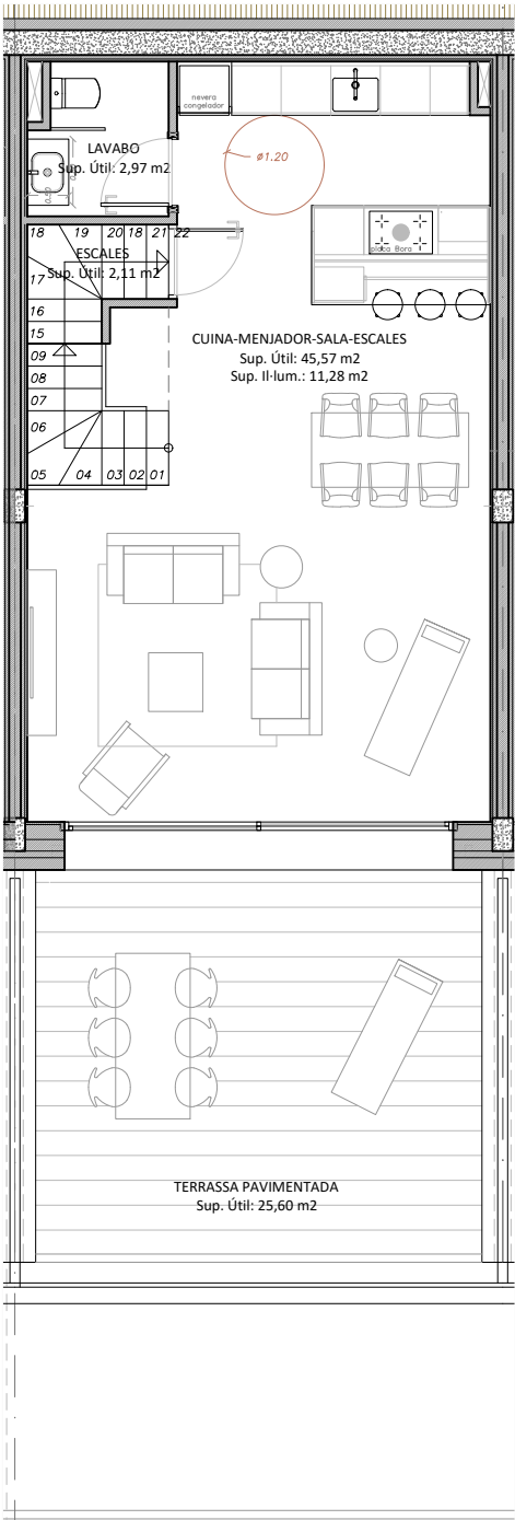
PLANTA BAIXA
