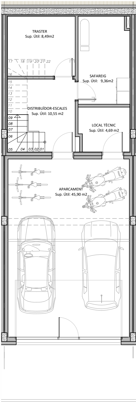
PLANTA SOTERRANI
