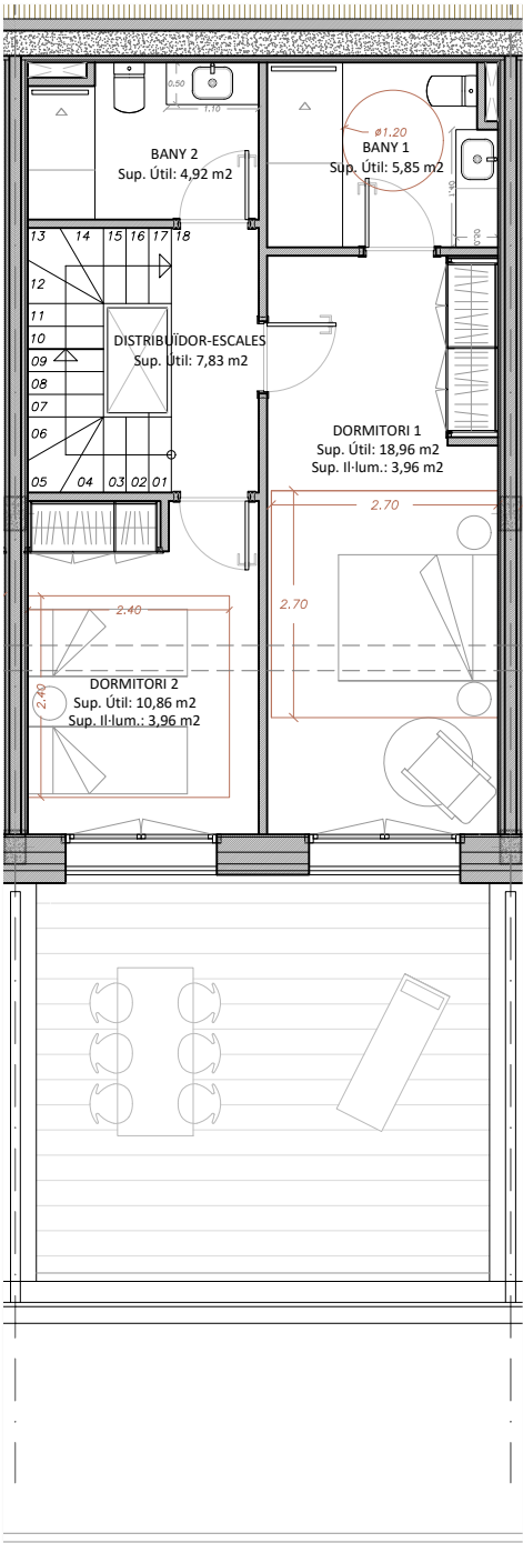
PLANTA PRIMERA
